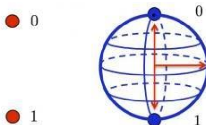
Рисунок 3. Классический Бит и Кубит
