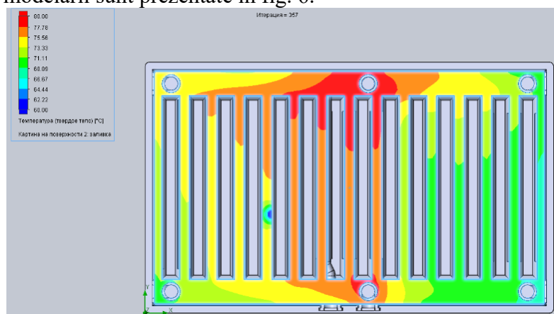
Figura 6. Дистрибуцiя температурi pe suprafaa radiatorului
