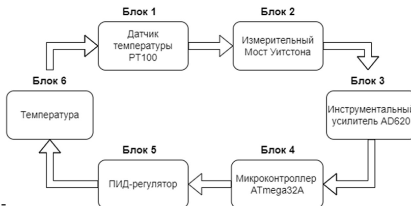
Рисунок 1. Блок-схема для считывания и регулирования температуры
